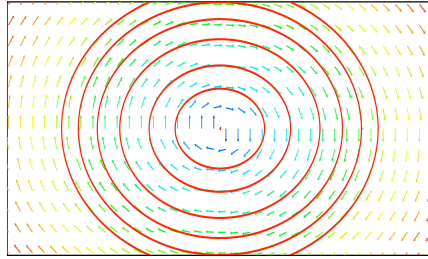
Retrato de fase do oscilador harmónico.
