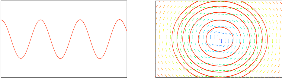
Uma trajectória e retrato de fases do oscilador harmónico.
