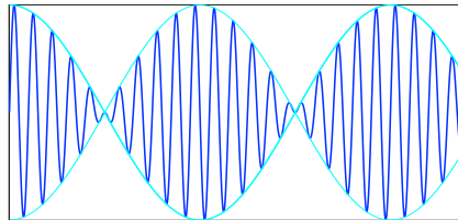
Sobreposição z(t) = \sin(0.95 \cdot t) + \sin(1.05 \cdot t) .
