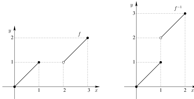
Figura 5.1: Função contínua com inversa descontínua. ■
