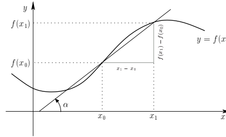
Figura 6.1: Interpretação geométrica da TVM_{[x_0, x_1]} .
