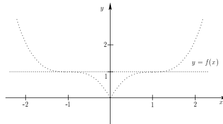
Figura 3.8: Função contínua exactamente em x = -1 e x = 1 . ■
