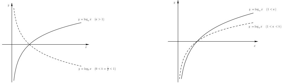
Figura 4.5: Esboços dos gráficos de funções logarítmicas.
